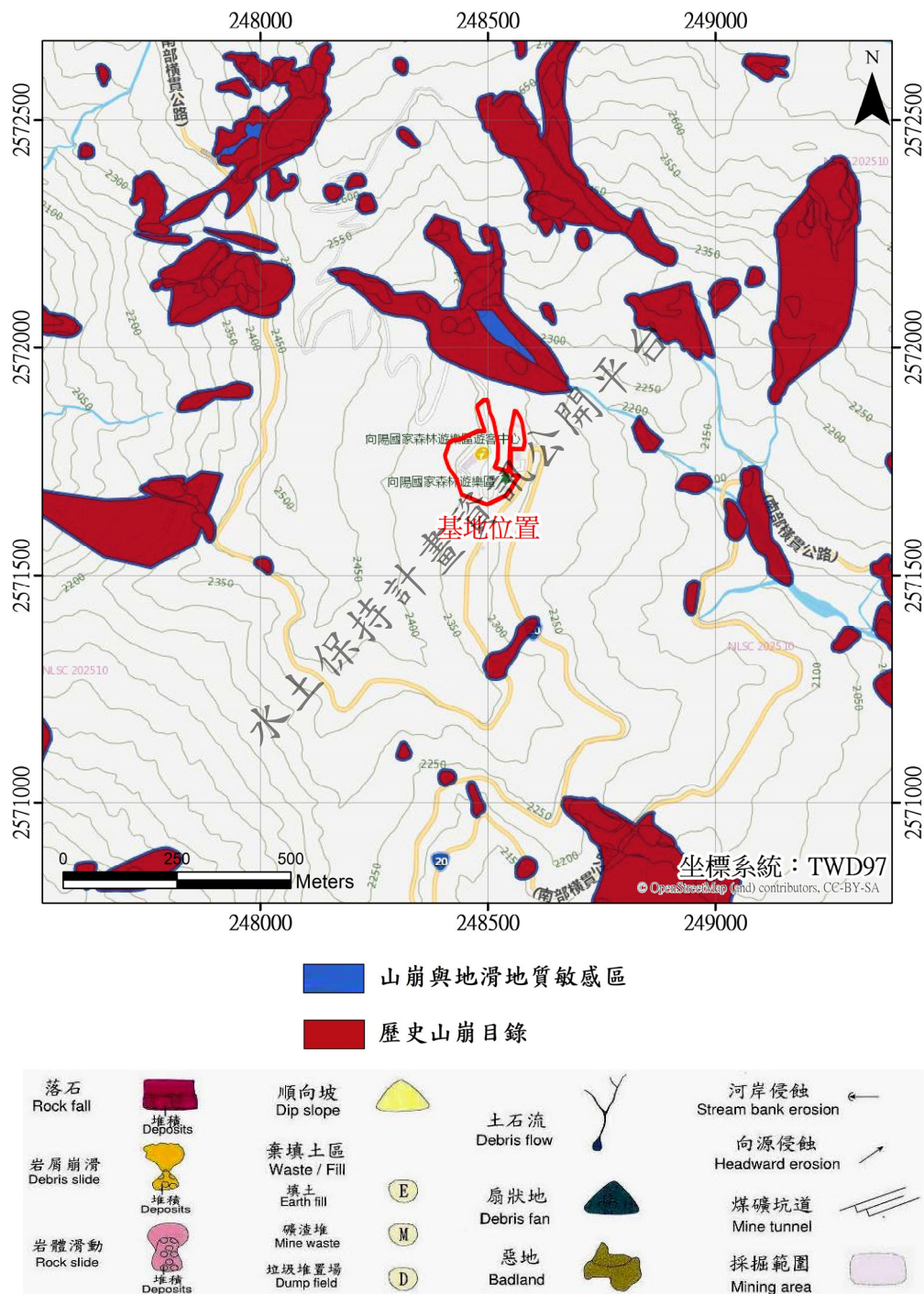
圖 4-0-6 環境地質圖
