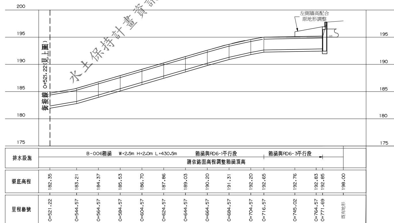
縱面圖 V=1:200 H=1:1,000
